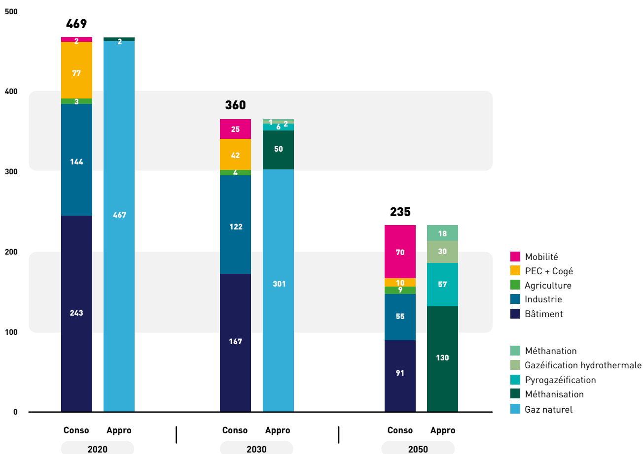
Consommations et approvisionnement de gaz en TWh PCS
