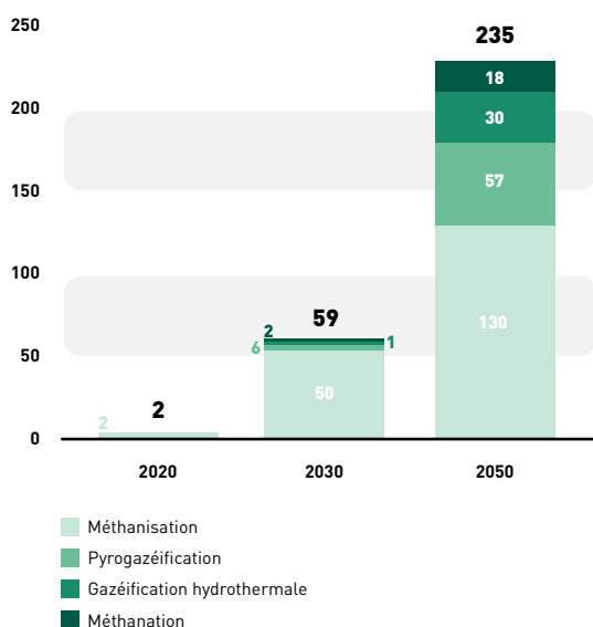
Production de méthane renouvelable et bas-carbone - TWh
